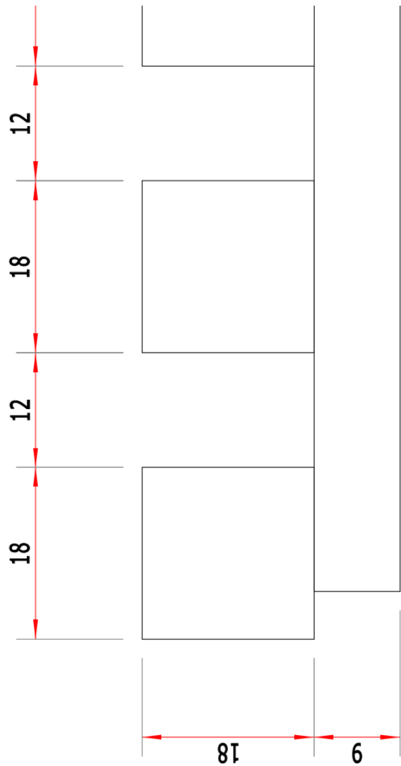
Doorsnede uiteinde
